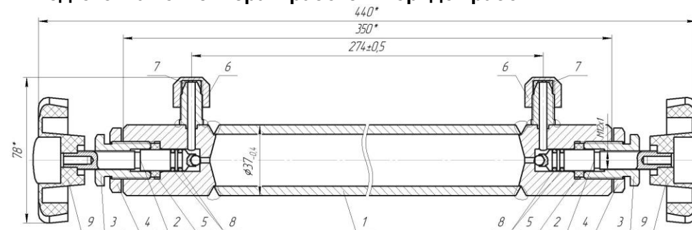
Рис.1 Контейнер для отбора проб КЖ-150: 1 – Корпус пробоотборника, 2 – Шток, 3 – Гайка, 4 – Гайка поджимная, 5 – Кольцо уплотнительное, 6 – Заглушка, 7 – Уплотнение заглушки, 8 – Уплотнение штока, 9 – Вороток.
